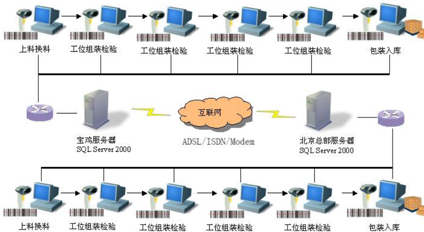
生产线条码管理系统网络结构示意图
